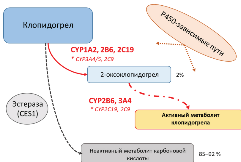
Рисунок 1. Краткая схема метаболизма клопидогрела.
